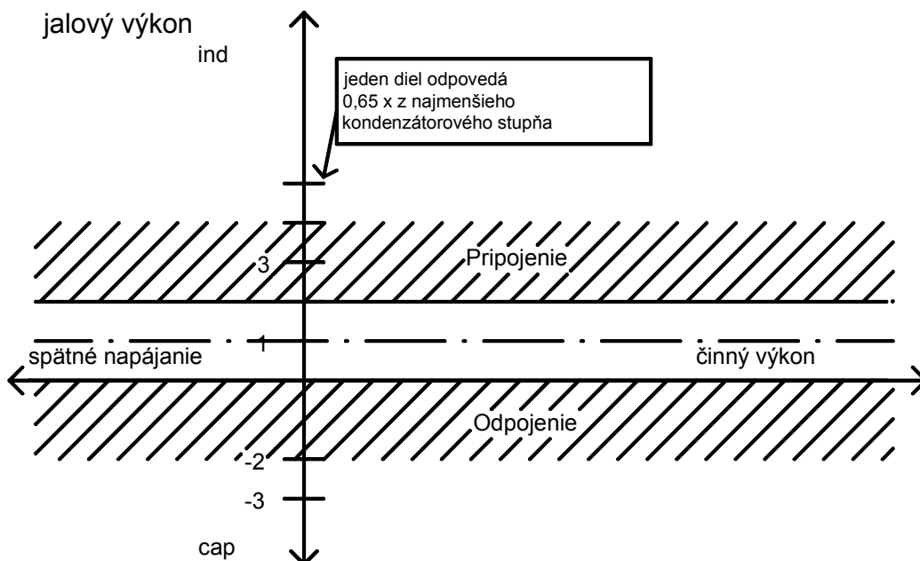
Obr. 6: Regulačné pásmo pri nastavení cieľového \cos \varphi = 1 ; L = \text{OFF} ; \text{PS} = +1,0
