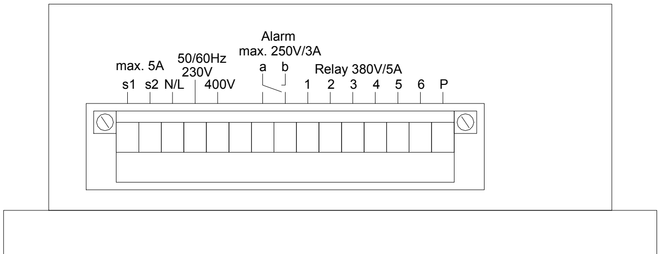
Obr. 2: Pohľad zospodu
