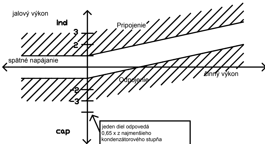
Obr. 5: Regulačné chovanie pri nastavení cieľového \cos \varphi = 0,92 ind.; L = \text{OFF} ; \text{PS} = 0
